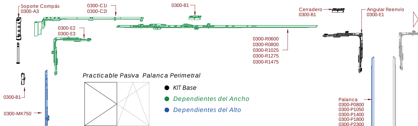
PRACTICABLE COTA VARIABLE - HOJA PASIVA - PALANCA PERIMETRAL - DERECHA/IZQUIERDA - HERRAJE ESTANDAR
