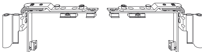
Falso Compás Izquierda Ref. 0300-JI
